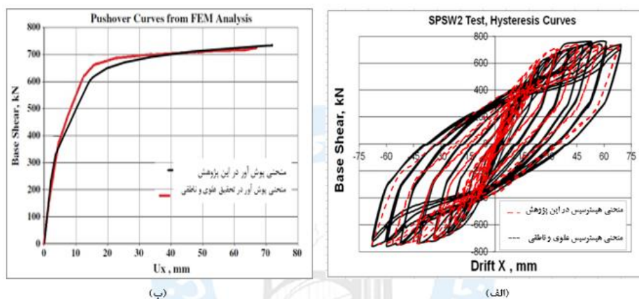
شکل ۸: مقایسه ی نمودارهای هیستریسیس (الف) و پوش آور (ب) مدل اجزاء محدودی این پژوهش با مدل ارائه شده در مقاله علوی و ناطقی
