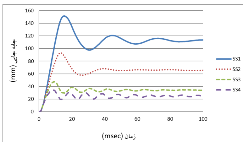
شکل ۱۴: نمودار تاریخچه زمانی تغییر مکان تراز بالای قاب در راستا X مدل های ساخته شده از ورق فولاد معمولی تحت اثر انفجار حوزه دور
