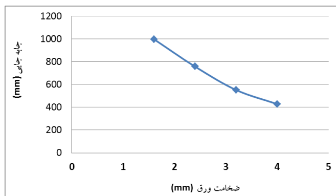
شکل ۱۳: تغییرات جابه جایی بالای دیوار برشی فولاد معمولی با تغییر ضخامت ورق تحت انفجار حوزه نزدیک
