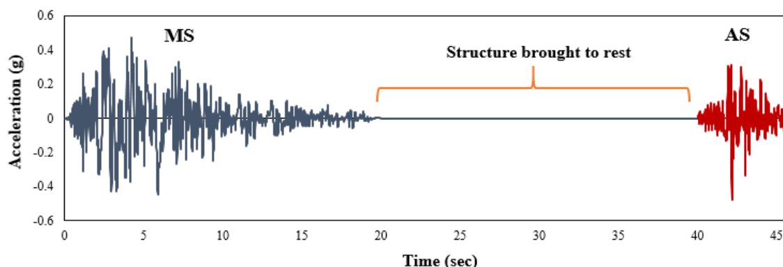
شکل ۴: تاریخچه زمانی شتاب حرکت زمین در یک توالی مورد استفاده قرار گرفته برای انجام تحلیل سازه‌های ۴ طبقه با سیستم RBRBF و BRBF (رکورد با شماره (RSN) ۱۰۶۳ به عنوان زلزله اصلی و رکورد با شماره (RSN) ۱۷۲۸ به عنوان پس‌لرزه).
