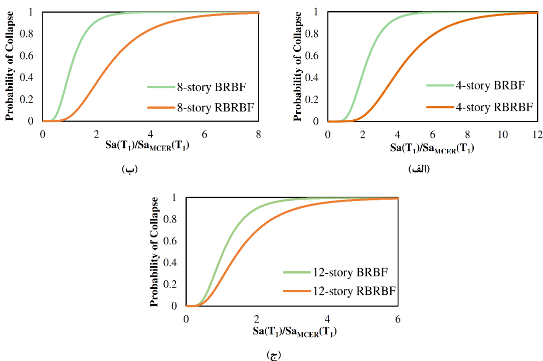
شکل ۱۰: مقایسه منحنی‌های شکنندگی فروریزش نرمال شده سازه‌های: الف) ۴ طبقه، ب) ۸ طبقه و ج) ۱۲ طبقه با سیستم‌های RBRBF و BRBF تحت Mainshock0.01+Aftershock0.1.
