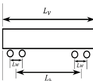
شکل ۹: هندسه یک واگن قطار پردیس، L_w طول یک واگن، L_b فاصله دو بوژی، L_y فاصله دو چرخ یک بوژی
