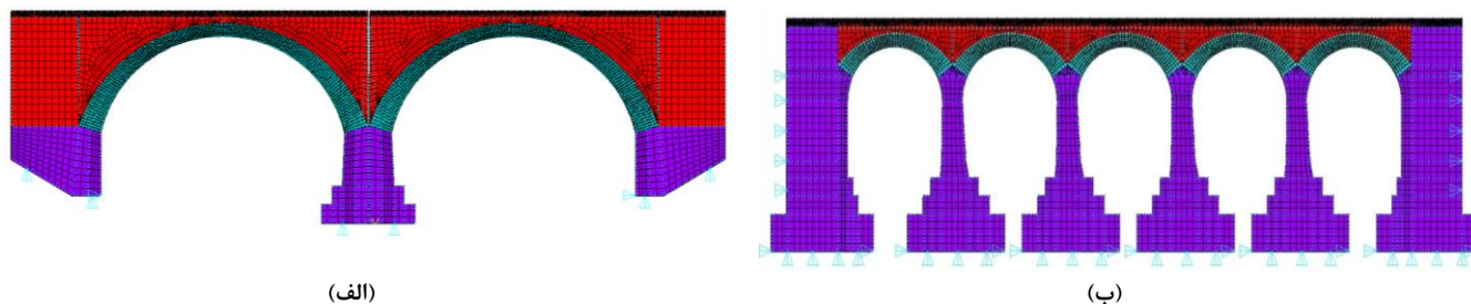
شکل ۲: مدل اجزای محدود و شرایط مرزی پل‌ها (الف) پل کیلومتر ۲۳ (ب) پل کیلومتر ۲۴
