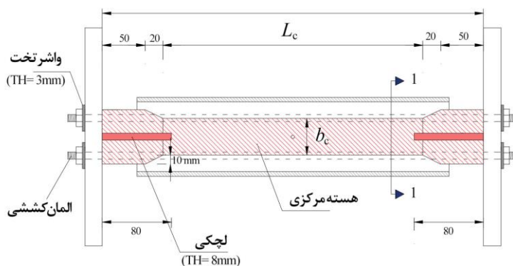
الف- جزئیات و ابعاد فیوز پیشنهادی (ابعاد به میلی متر)
