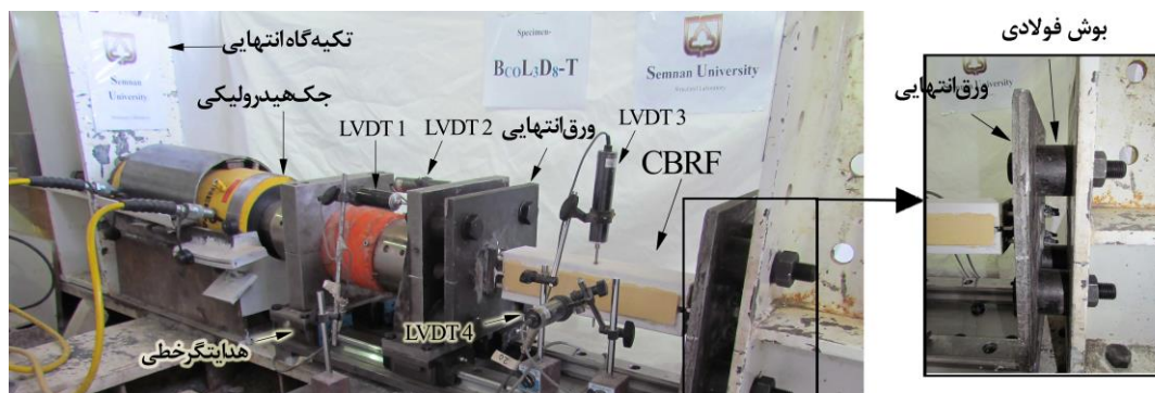
شکل ۶: پیکربندی آزمایش
