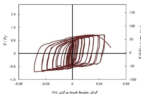
الف- نمودار هیستریزس RL-BRB
