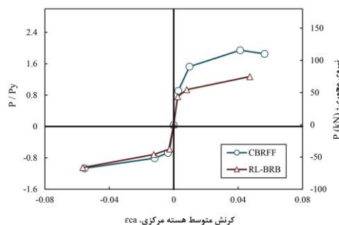
الف- مقایسه منحنی‌های برازش شده هیستریزس
