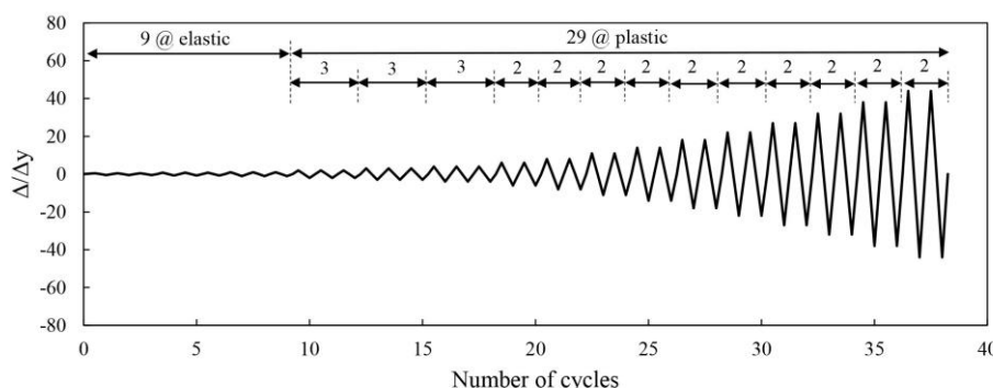
شکل ۵: پروتکل بارگذاری
