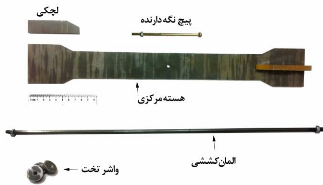
ج- جزئیات ساخته شده فیوز
