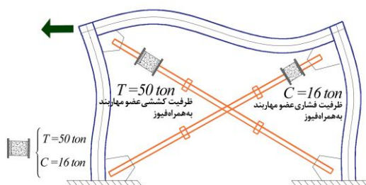
د- ظرفیت باربری مهاربند ضمن استفاده از CBRF
