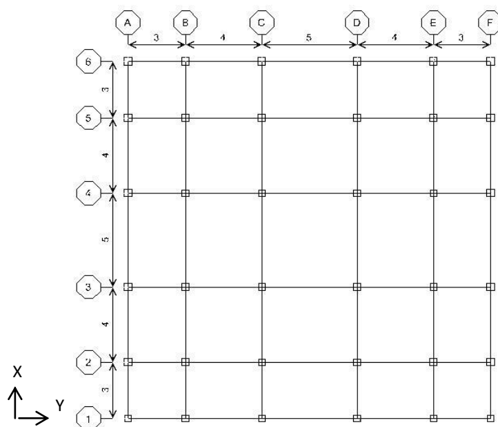
شکل ۱: پلان مدل‌ها (اندازه‌ها بر حسب متر).
