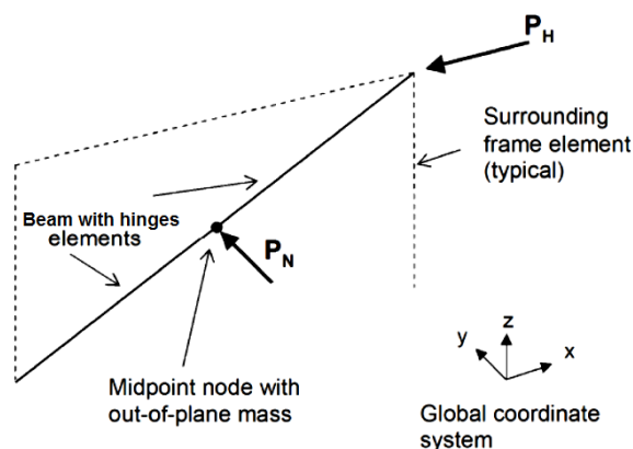
شکل ۴: دستک فشاری قطری معادل [۲۹].
