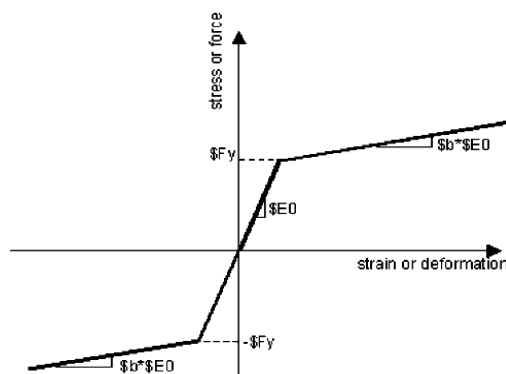
شکل ۶: رفتار تنش-کرنش مصالح تک محوری Steel01 [۱۹].
