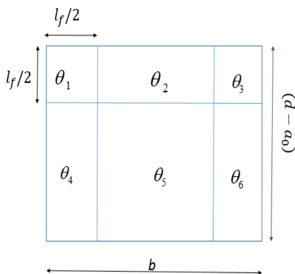
شکل ۵: فاکتور جهت بر اساس تقسیم بندی Dupont و Vandewall
