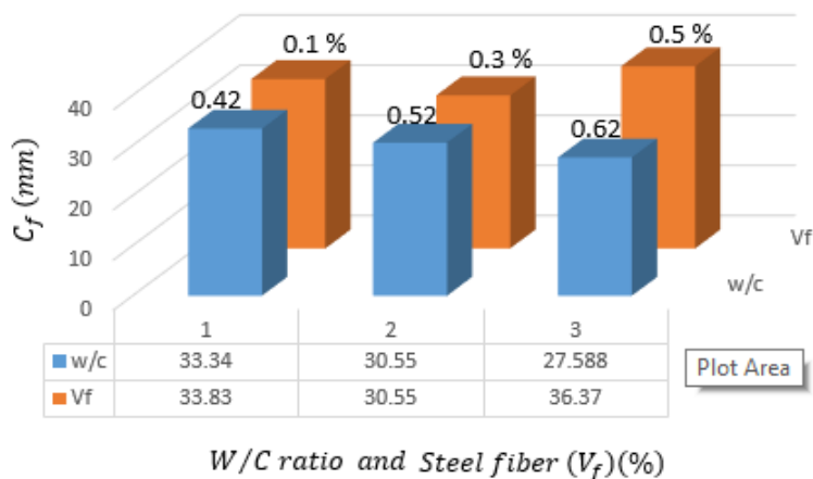
شکل ۹: پارامتر طول منطقه صدمه دیده نوک ترک به روش اثر اندازه برای نسبت های آب به سیمان مختلف و درصد الیاف فولادی
