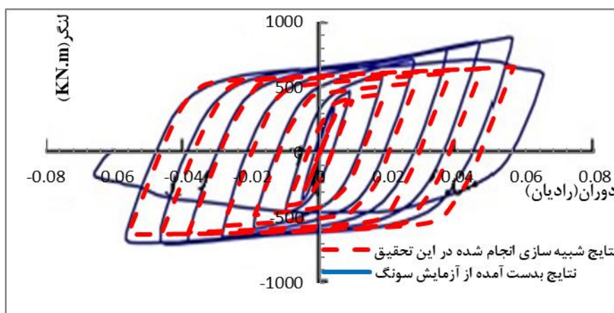
شکل ۴: مقایسه بین منحنی هیستریزیس به دست آمده از نتایج آزمایشگاهی سونگ و شبیه‌سازی انجام شده در این تحقیق.
