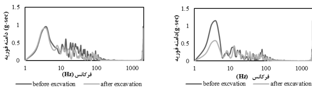
ب- نقطه شماره ۵ واقع بر دیوار گود
