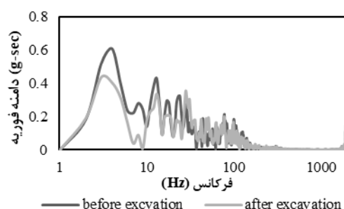
الف - نقطه ۶ شماره واقع بر کف گود
