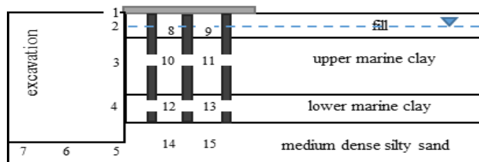
شکل ۶: شماره‌گذاری نقاط انتخاب شده در مدل اول و سوم.
