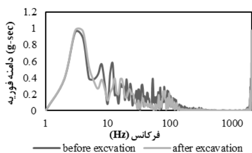
ب - نقطه شماره ۳ واقع بر دیوار گود
