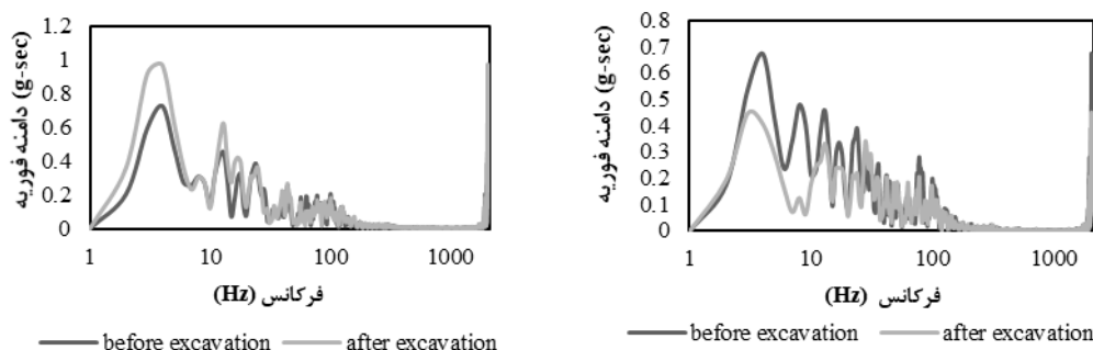
ب - نقطه شماره ۲ واقع در لایه چهارم
