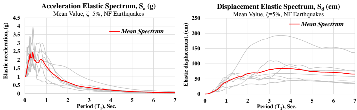
شکل ۴: نمودار طیف الاستیک شتاب و تغییر مکان زلزله‌های حوزه نزدیک (هر رکورد و میانگین آن‌ها)
