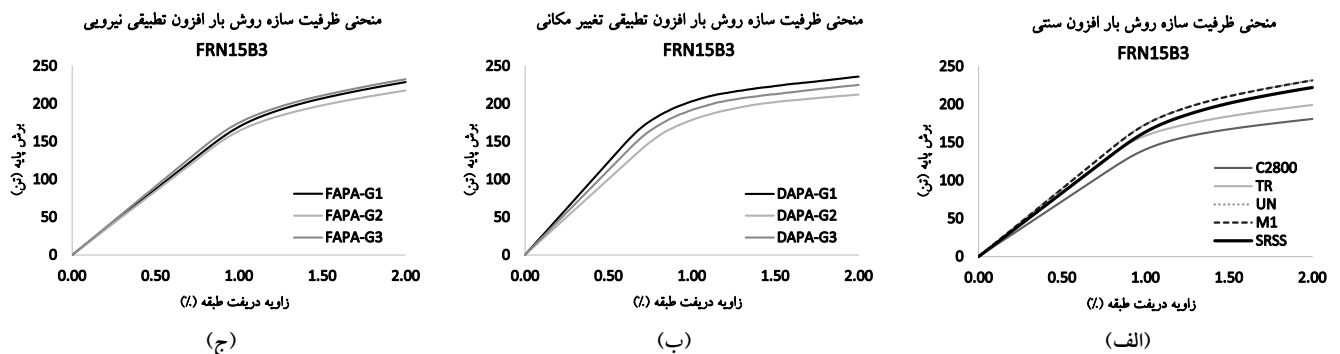
شکل ۷: منحنی ظرفیت برای قاب FRN15B3: (الف) روش CPA، (ب) روش DAPA، (ج) روش FAPA
