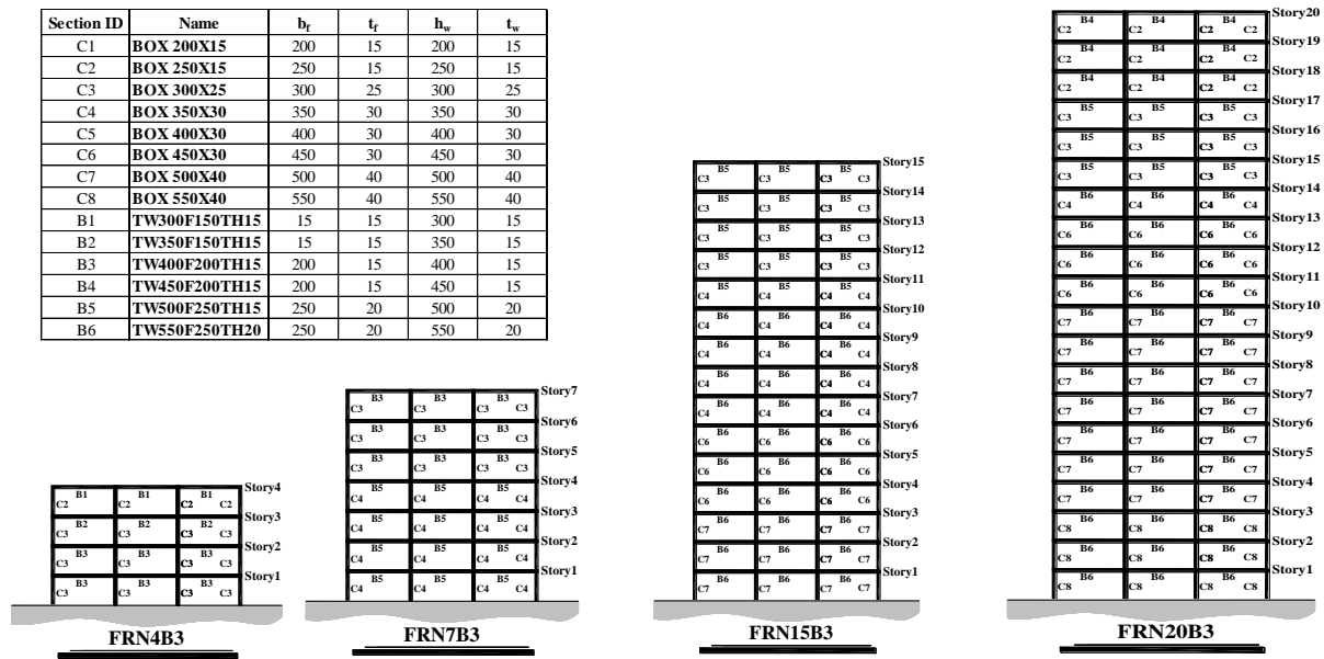
شکل ۳: جزییات مدل‌های سازه‌ای مورد استفاده در فرآیند تحلیل بار افزون و تاریخچه زمانی
