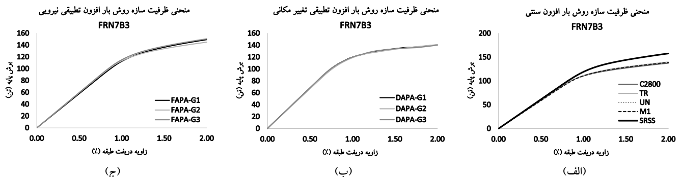
شکل ۶: منحنی ظرفیت برای قاب FRN7B3: (الف) روش CPA، (ب) روش DAPA، (ج) روش FAPA
