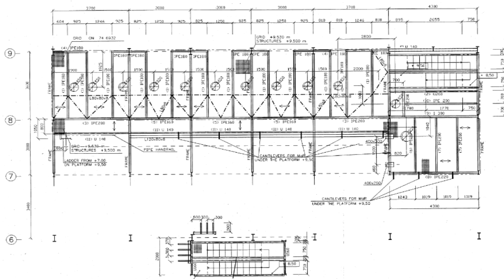
شکل ۱: نمونه نقشه سوله فولادی
