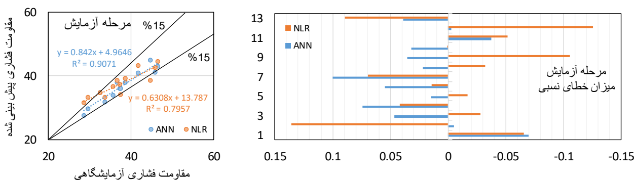
شکل ۱۱: نمودار پراکندگی برای پیش بینی مقاومت فشاری بتن ژئوپلیمر در مرحله آزمایش
