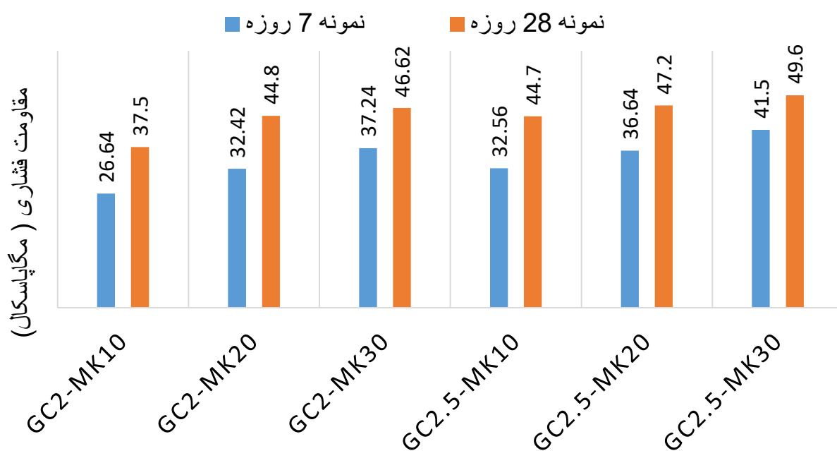
شکل ۳: تاثیر نسبت \text{NaOH}/\text{Na}_2\text{SiO}_3 بر مقاومت فشاری ۷ و ۲۸ روزه بتن
