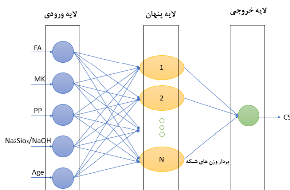
شکل ۹: معماری شبکه روش ANN برای مدل سازی مقاومت فشاری بتن ژئوپلیمر
