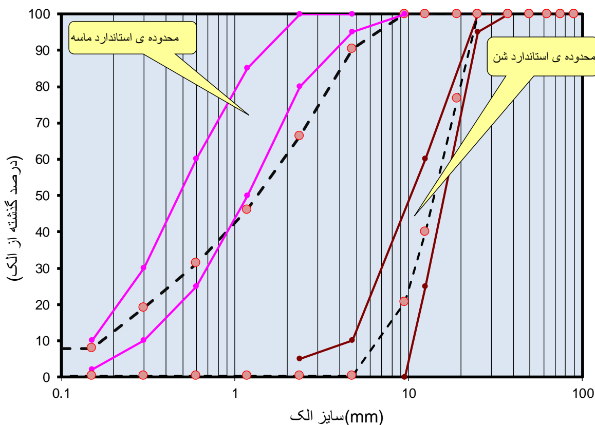
شکل ۱: نمودار دانه‌بندی مصالح سنگی بازیافتی
