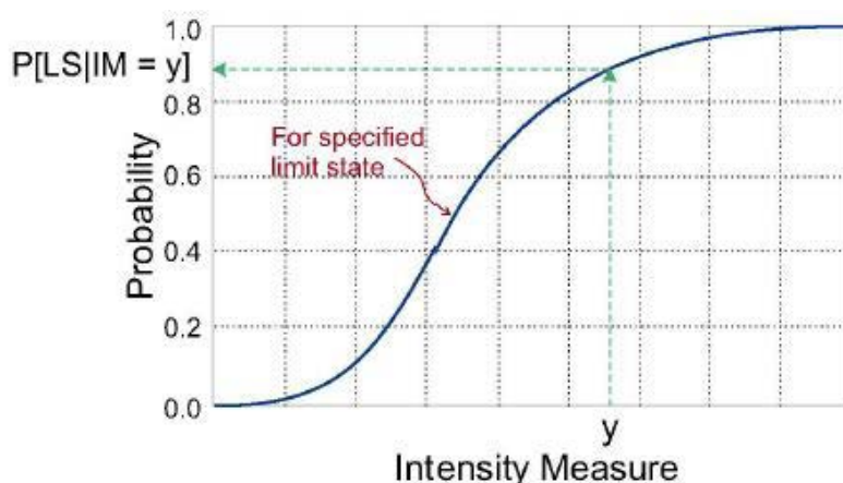
شکل ۲: فرم کلی منحنی‌های شکنندگی [۴]
