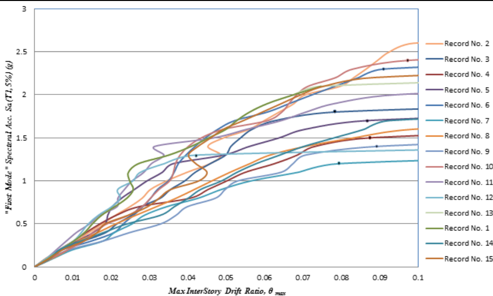
شکل ۷: منحنی های IDA بدست آمده برای قاب سازه ای ۴ طبقه دارای مهاربند شورون با میراگر ویسکوز
