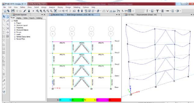
شکل ۵: فایل مدل سازی شده به شکل دو بعدی برای سازه ۴ طبقه دارای مهاربند شورون در نرم افزار ایتبز ۲۰۱۵
