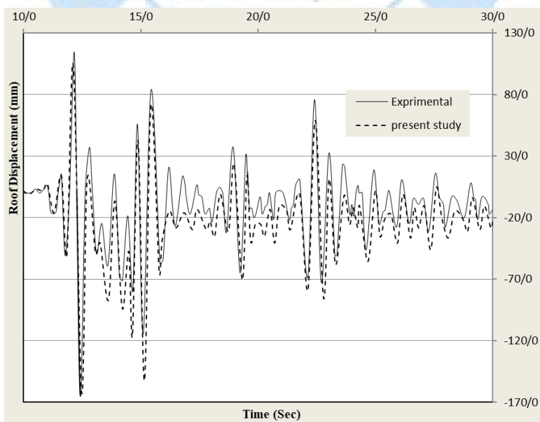
شکل ۱۵: مدل سازی تغییرمکان بام برای سازه مقاوم سازی شده تحت زلزله ال سنترو (۰.۲۷۵٪) و مدل مطالعه حاضر
