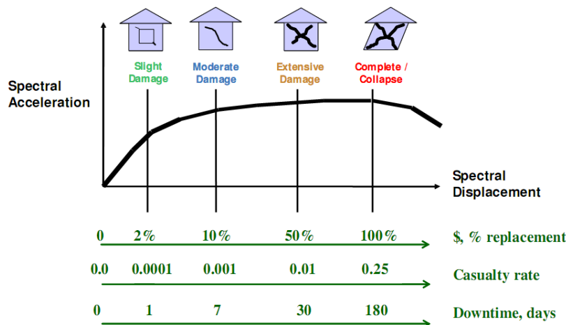
شکل ۳: توابع خسارت ساختمان [۵]
