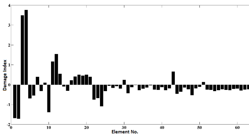
شکل ۷: اندیس آسیب المان‌ها در حالت خرابی شماره ۵ با اعمال ۱۵ درصد آسیب
