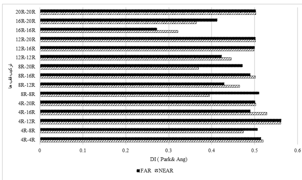
شکل ۷: میانگین شاخص خسارت طبقات در میانگین رکوردهای حوزه نزدیک و دور از گسل در ترکیب قاب‌های منظم - منظم
