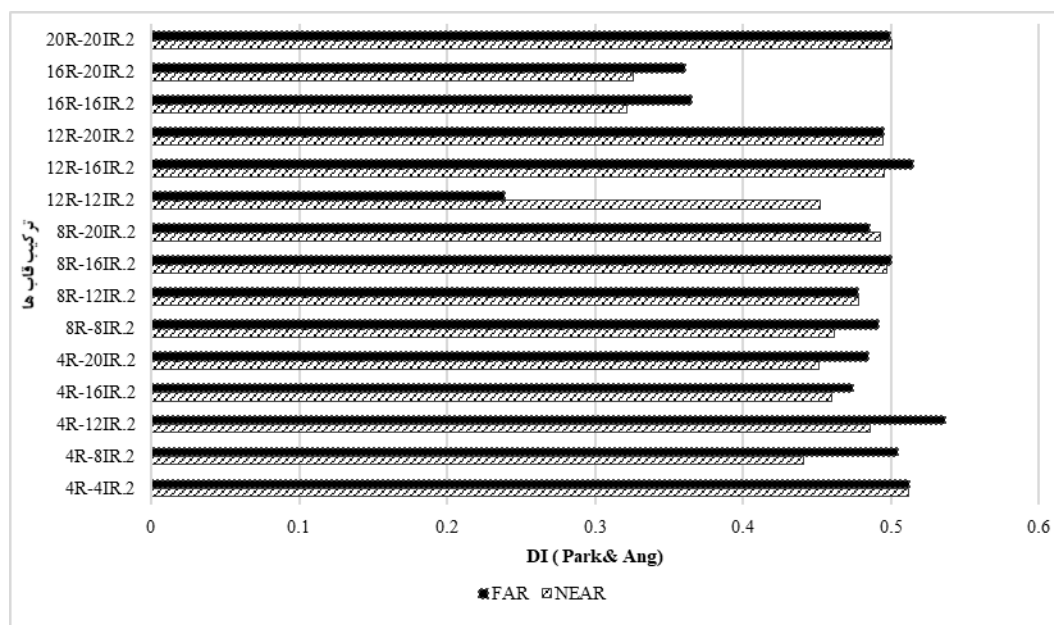
شکل ۹: میانگین شاخص خسارت طبقات در میانگین رکوردهای حوزه نزدیک و دور از گسل در ترکیب قاب‌های منظم - نامنظم نوع ۲
