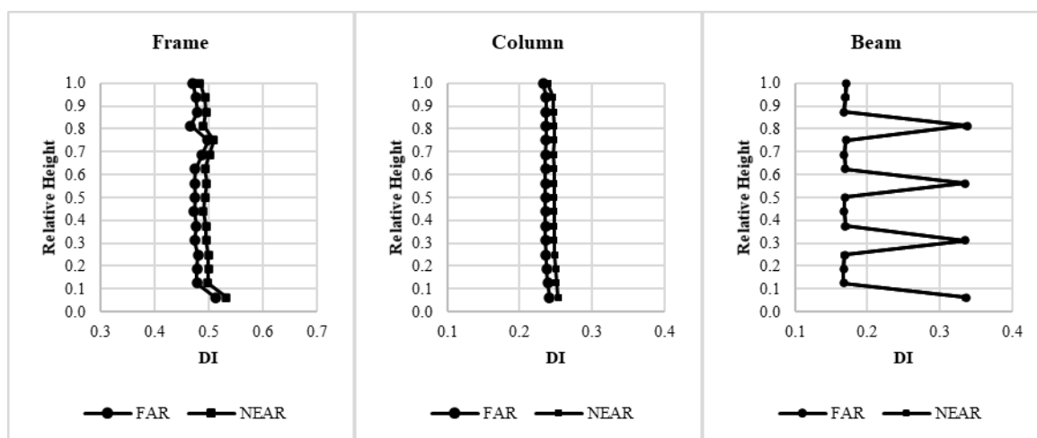
ج) مقایسه شاخص خسارت کل طبقه در طبقات قاب ۱۶ طبقه منظم
