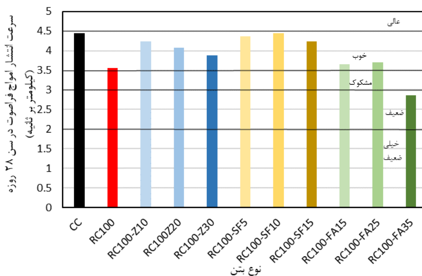
نمودار شماره ۶- سرعت امواج فراصوت در انواع بتن‌های معمولی و بازیافتی
