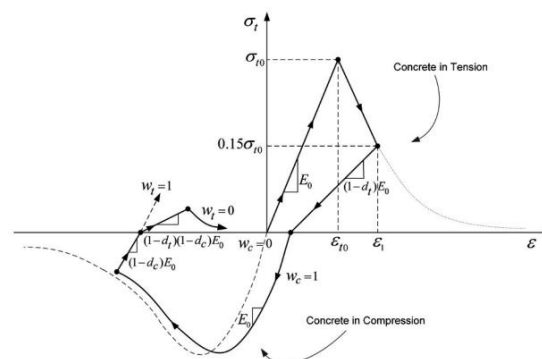
(الف) منحنی رفتار بتن در فشار و کشش
