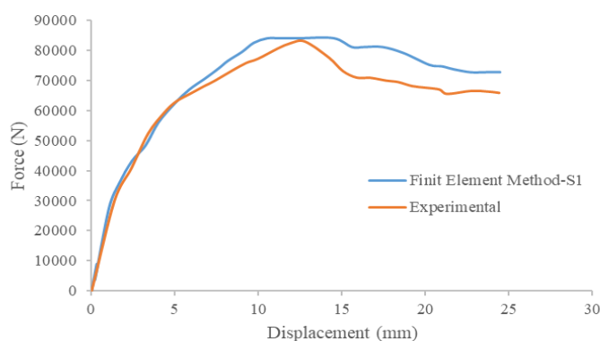
شکل ۹- منحنی بار تغییرمکان تیر ساده تحت اثر بار برای محاسبه برش
