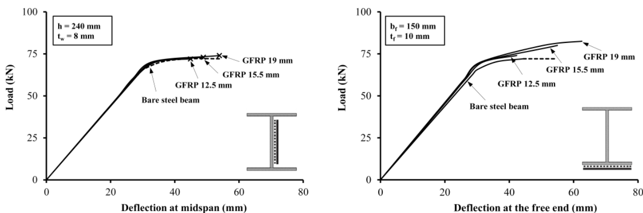
شکل ۱۷: نمودار بار-تغییر مکان انتهای آزاد Beam1 یک سر گیردار در حالت چیدمان ورق GFRP بر روی بال فشاری و جان
