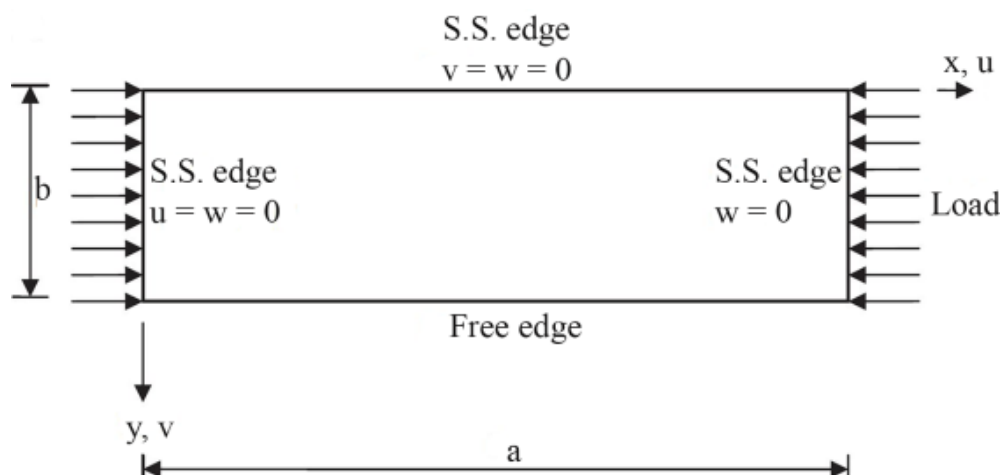
شکل ۴: شرایط مرزی به صورت تکیه‌گاه مفصلی در سه لبه و یک لبه آزاد برای ورق فولادی تحت فشار در تحقیق الصدیقی و الداماتی [۱۳]
