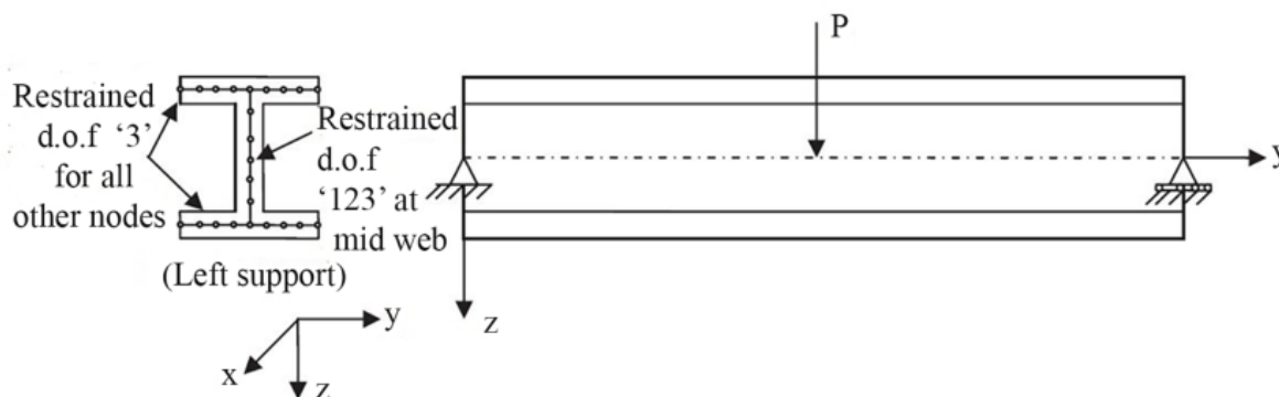
شکل ۷: نحوه اعمال شرایط مرزی و بارگذاری تیر دو سر مفصل [۱۱]
