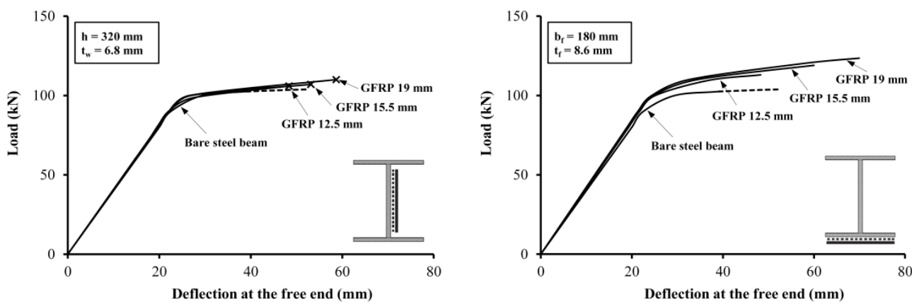
شکل ۱۸: نمودار بار-تغییر مکان انتهای آزاد Beam2 یک سر گیردار در حالت چیدمان ورق GFRP بر روی بال فشاری و جان
