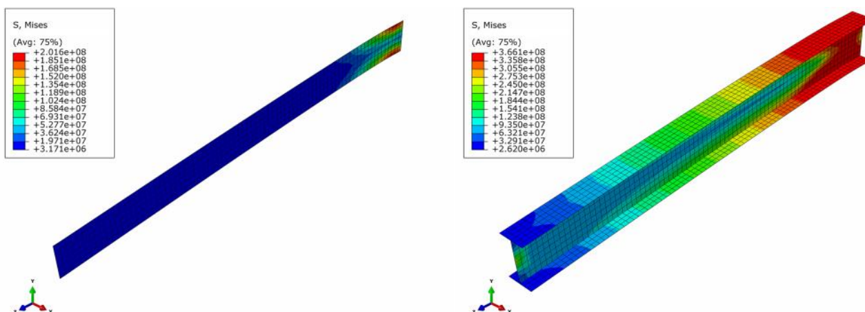
شکل ۲۰: حالت توزیع تنش در تیر فولادی و ورق GFRP برای نمونه Beam1 یک سر گیردار در حالت چیدمان ورق GFRP بر روی جان
