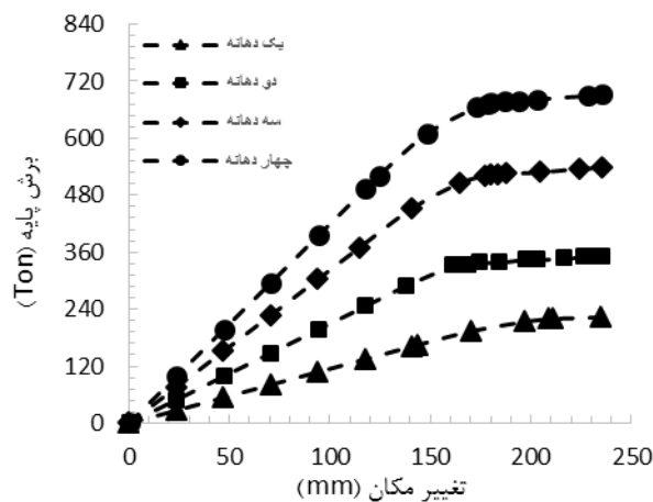
(د) سازه ۶ طبقه، الگوی بار (UEY)
