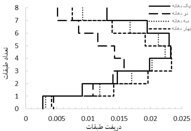
ج) سازه ۸ طبقه، الگوی بار (TEY)، ضریب نامعینی ۱,۲
