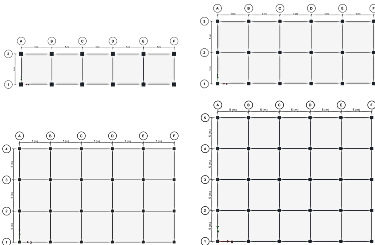
شکل ۵: پلان ساختمان های مورد مطالعه
