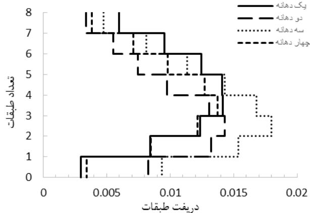
د) سازه ۸ طبقه، الگوی بار (UEY)، ضریب نامعینی ۱,۲
