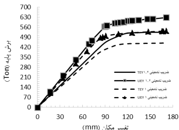
(ج) چهار دهانه
