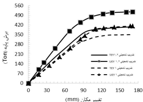
(د) سه دهانه
