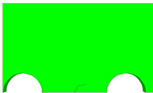
شکل ۱۲: مسیر انتشار ترک با زاویه اولیه ۶۰ درجه برای رشد ۳ میلیمتر.
