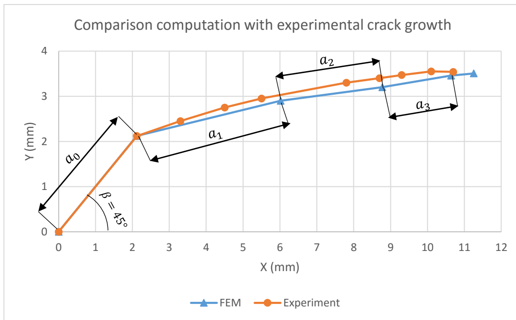
شکل ۹: نمودار مقایسه ی مسیر رشد ترک به روش FE با روش تجربی ماریجا بلازیک و همکاران [۶].
