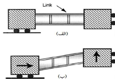
شکل ۲: اعمال شرایط مرزی. الف) مدل در حالت اولیه ب) مدل در حالت تغییر شکل یافته [۲۱]
