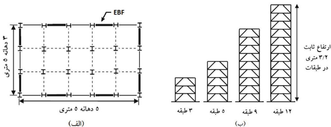
شکل ۴: نمای مدل‌های مورد بررسی در این مطالعه. الف) پلان سازه ب) نمای جانبی قاب‌ها
