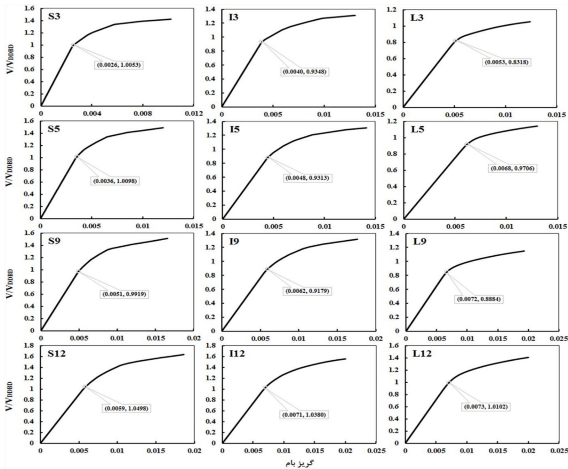
شکل ۵: منحنی ظرفیت قاب‌های واگرای ۳، ۵، ۹ و ۱۲ طبقه با انواع عملکرد تیر پیوند
