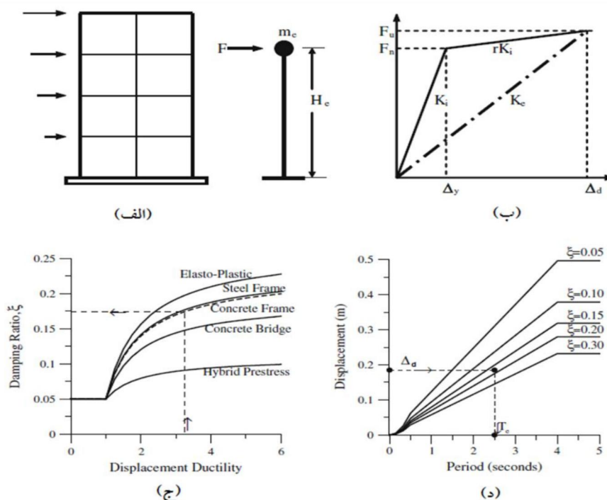
شکل ۱: مراحل روش طراحی مستقیم بر مبنای تغییرمکان. الف) معادل‌سازی سیستم یک درجه آزادی (ب) سختی مؤثر K_e (ج) میرایی معادل در مقابل شکل‌پذیری (د) طیف تغییرمکان طراحی [۵]
