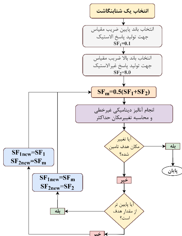
شکل (۳): فلوچارت روند تغییر در ضریب مقیاس
