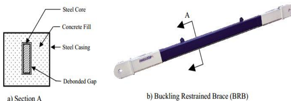
شکل ۱: قسمت‌های تفکیک شده‌ی مهاربند کمانش ناپذیر [۶].
