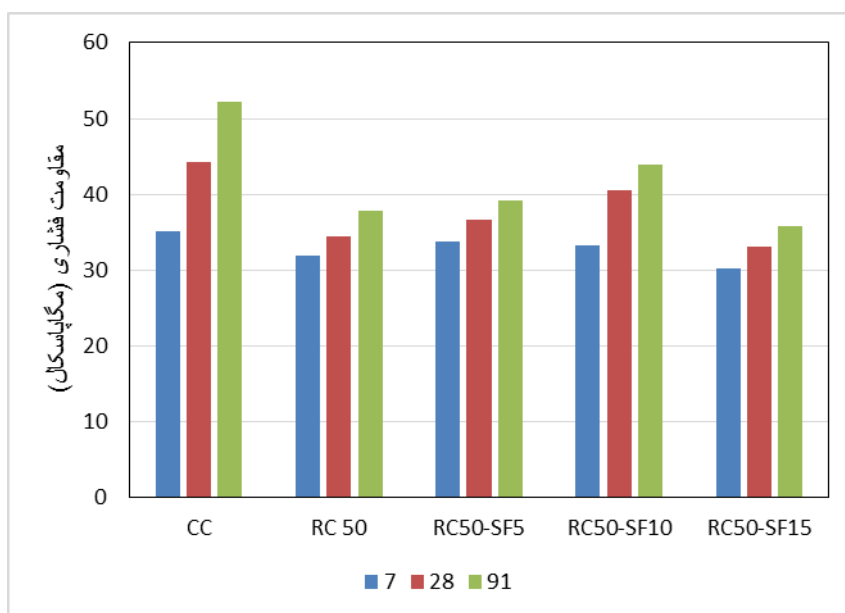
نمودار ۲: تغییرات مقاومت فشاری بتن‌های دارای ۵۰٪ ریزدانه بازیافتی
