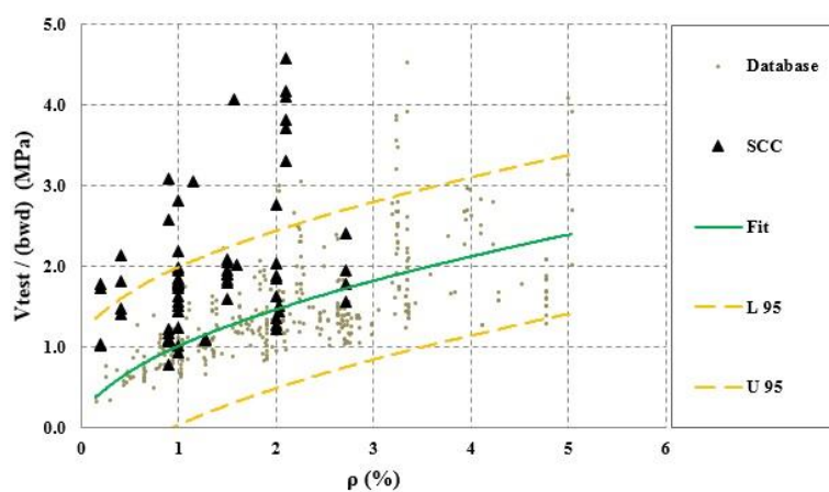
شکل ۳: مقایسه داده‌های مقاومت برشی بتن خودتراکم با بتن معمولی (تنش برشی - درصد فولاد طولی)
