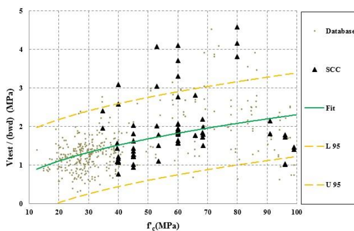
شکل ۴ - مقایسه داده‌های مقاومت برشی بتن خودتراکم با بتن معمولی (تنش برشی - مقاومت فشاری)
