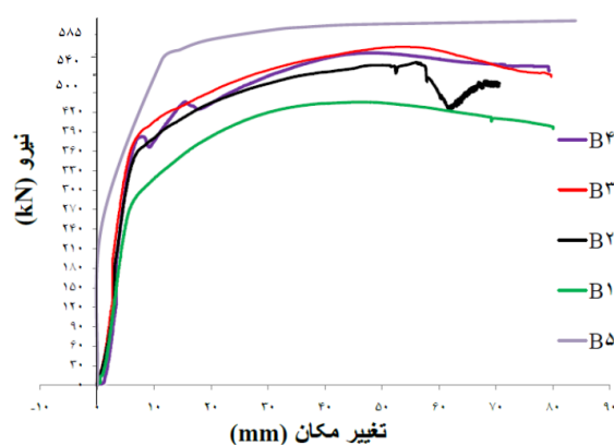
شکل ۶: نمودار نیرو-تغییر مکان محوری نمونه ها
