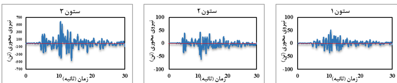
شکل ۲۲: تاریخچه زمانی نیروی محوری ستون‌های طبقه اول سازه (شکل ۸) با سیستم دوگانه قاب خمشی - پانل‌های شورون معکوس تحت رکورد طبس.
