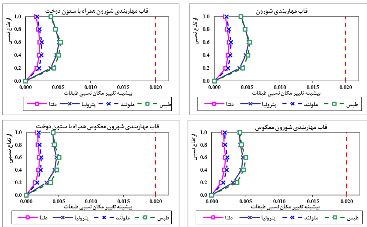
شکل ۱۵: نمودار پوش تغییر مکان نسبی (دریفت) راستای Y چهار سازه ۵ طبقه مطالعاتی؛ شامل سیستم دوگانه ترکیبی قاب خمشی و چهار ساختار جداگانه پانل‌های شورون، شورون همراه با ستون دوجت، شورون معکوس و نیز شورون معکوس همراه با ستون دوجت.
