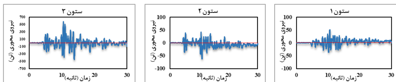
شکل ۲۳: تاریخچه زمانی نیروی محوری ستون‌های طبقه اول سازه (شکل ۸) با سیستم دوگانه قاب خمشی - پانل‌های شورون معکوس همراه با ستون دخت تحت رکورد طبس.
