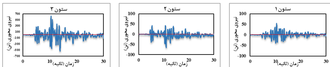
شکل ۲۱: تاریخچه زمانی نیروی محوری ستون‌های طبقه اول سازه (شکل ۸) با سیستم دوگانه قاب خمشی - پانل‌های شورون همراه با ستون دخت تحت رکورد طبس.
