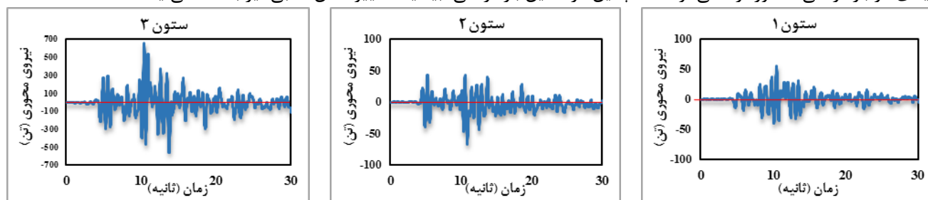
شکل ۲۰: تاریخچه زمانی نیروی محوری ستون‌های طبقه اول سازه (شکل ۸) با سیستم دوگانه قاب خمشی - پانل‌های شورون تحت رکورد طبس.
