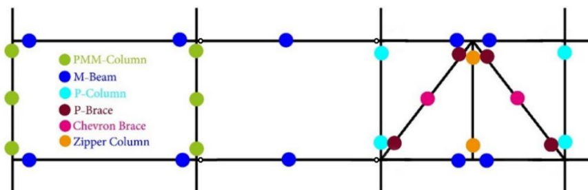
شکل ۱۰: آرایش قرارگیری مفصل احتمالی غیرخطی در المان‌های سازه‌ای مدل‌های مطالعاتی؛ پانل سمت راست از نوع مهاربندی شده و دارای المان ستون دوخت است و پانل سمت چپ از نوع خمشی می‌باشد [۲۷]
