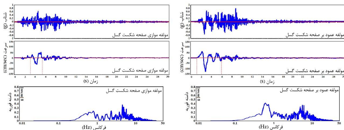
شکل ۳: تاریخچه زمانی شتاب، سرعت و طیف فوریه متناظر با دو مولفه افقی موازی و عمود بر صفحه شکست گسل رکورد بم ۲۰۰۳ میلادی؛
