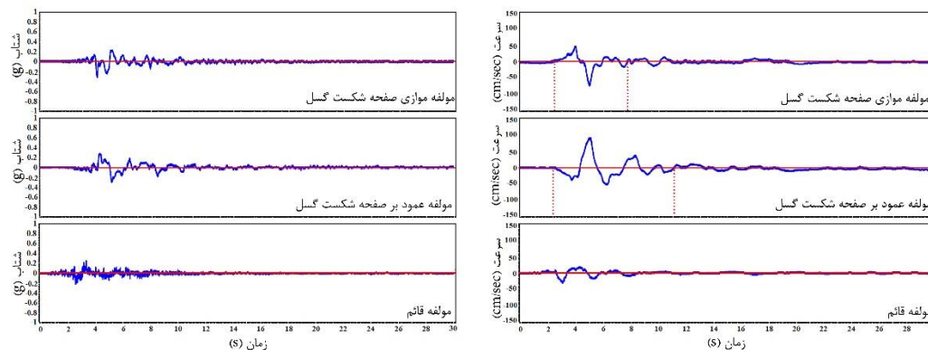
شکل ۵: تاریخچه زمانی سه مولفه شتاب و سرعت رکورد ملولند اورپس ثبت شده در زلزله امپریال ولی ۱۹۷۹؛
