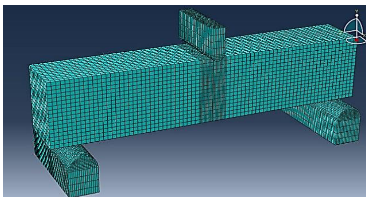
شکل ۵: مش‌بندی مدل اجزای محدود
