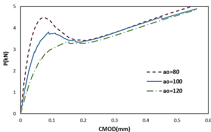
شکل ۱۴: نمودار بار-بازشدگی دهانه ترک برای طول ترک اولیه متغیر.
