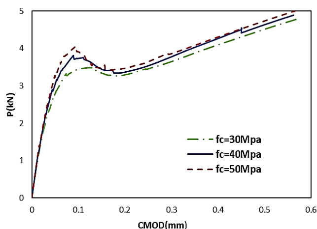
شکل ۹: نمودار بار-بازشدگی دهانه ترک برای تیرهایی با مقاومت ۳۰، ۴۰ و ۵۰ مگاپاسکال.
