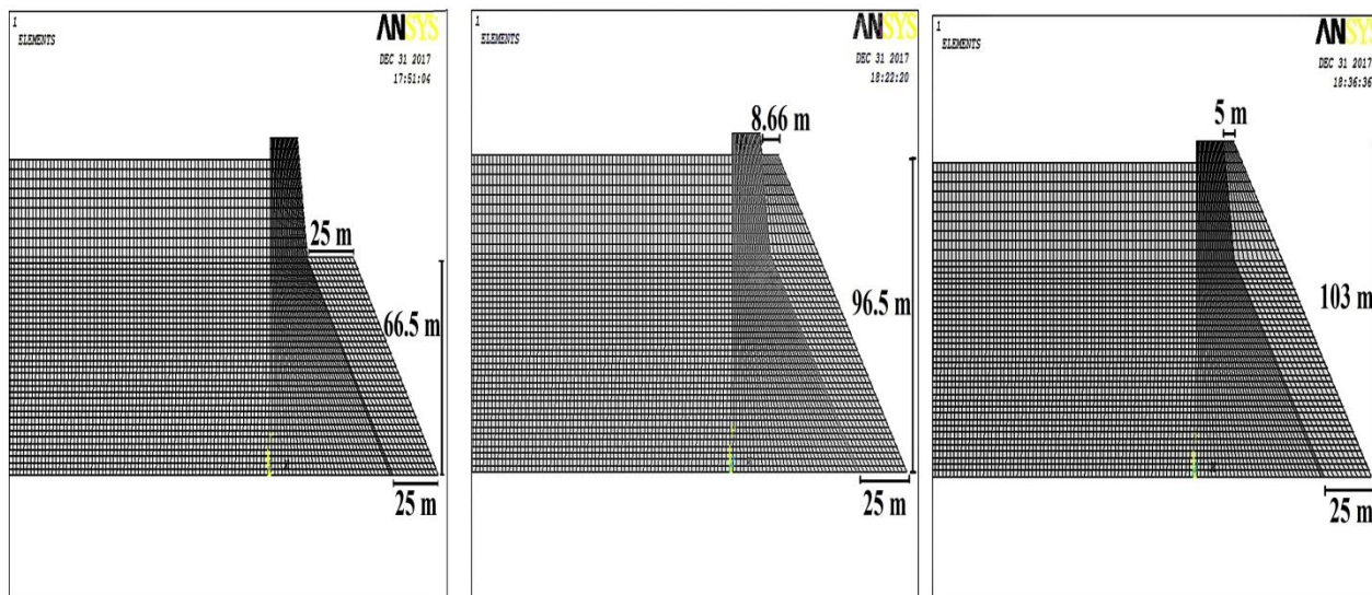
شکل ۴: مدل‌های پیشنهادی سیستم دارای حائل نگهدارنده آسفالتی
