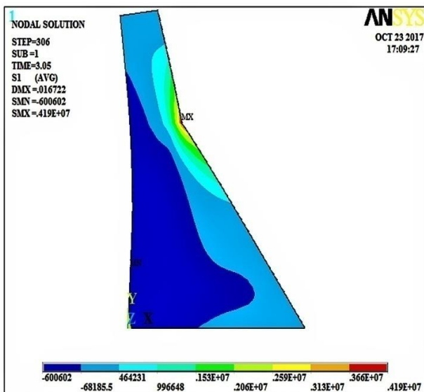
شکل ۱۲: کانتور تنش اصلی اول ( t=3.05\text{sec} )
