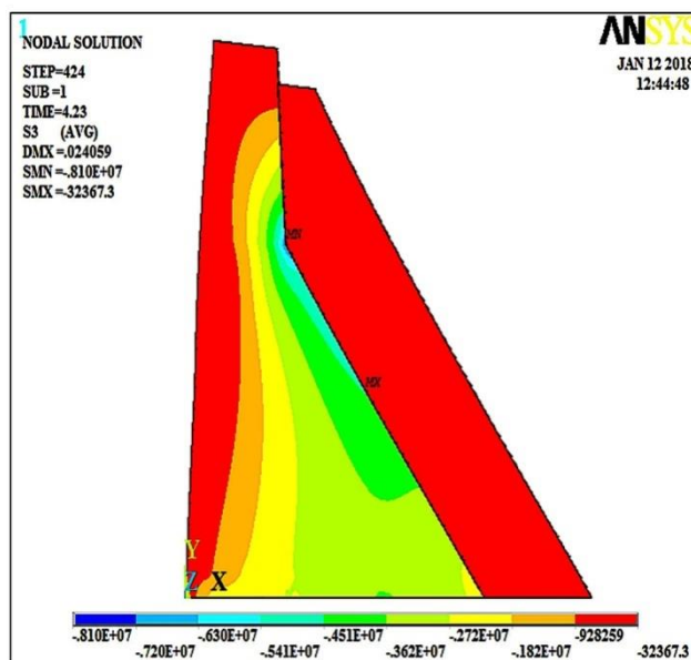
شکل ۲۰: کانتور تنش اصلی اول (t=4.33sec)
