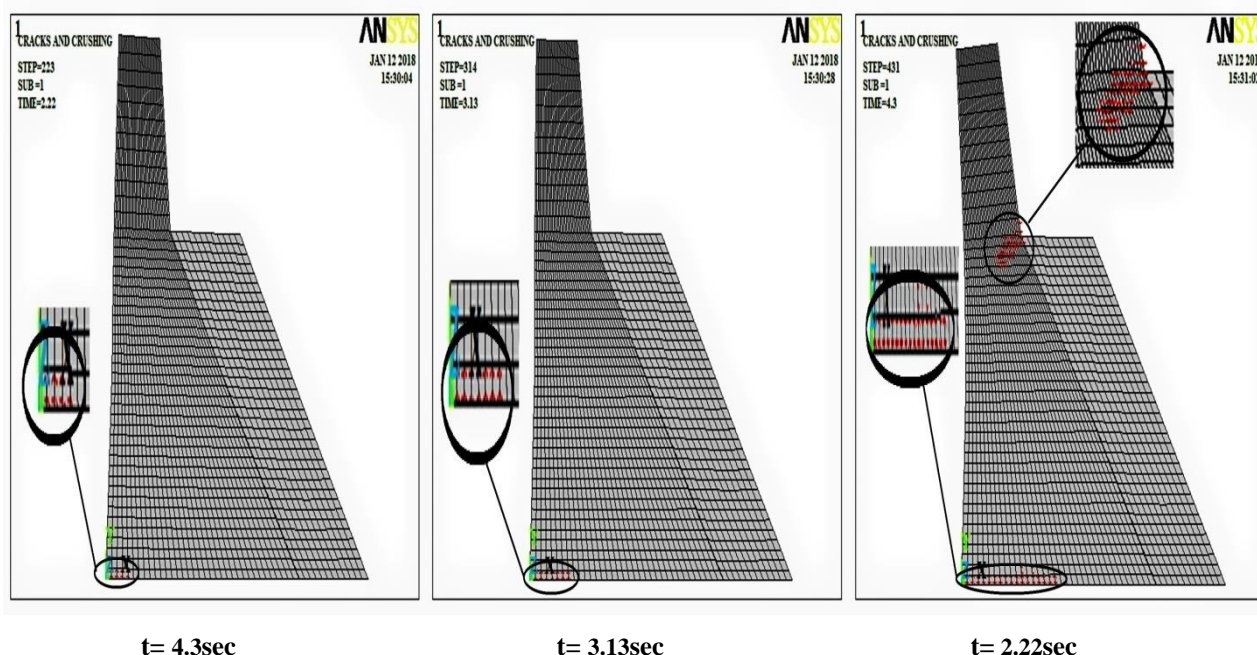
شکل ۳۳: الگوی رشد ترک در سد کوینا دارای حائل نگهدارنده‌ی آسفالتی 66.5 متری
