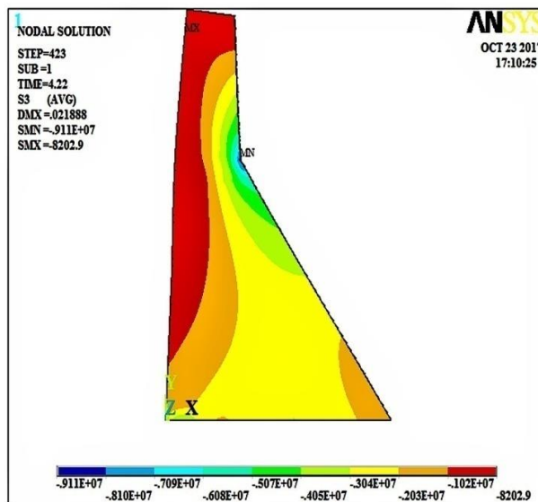
شکل ۱۳: کانتور تنش اصلی سوم ( t=4.22\text{sec} )
