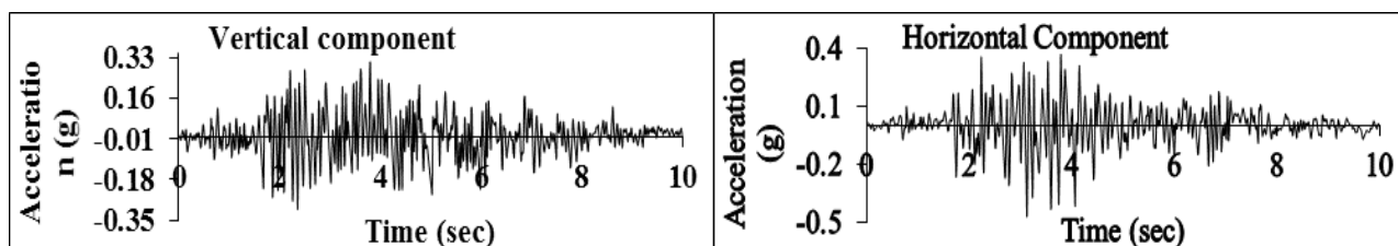
شکل ۶: مؤلفه‌ی افقی وقائم شتاب‌نگاشت زلزله Koyna
