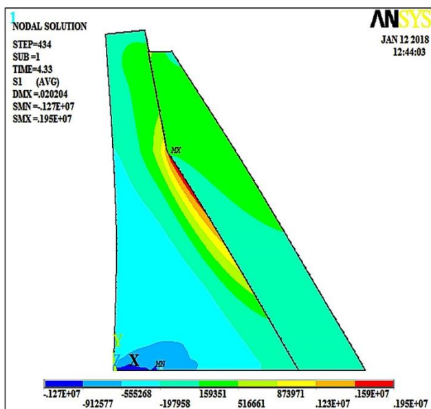
شکل ۲۱: کانتور تنش اصلی سوم (t=4.23sec)
