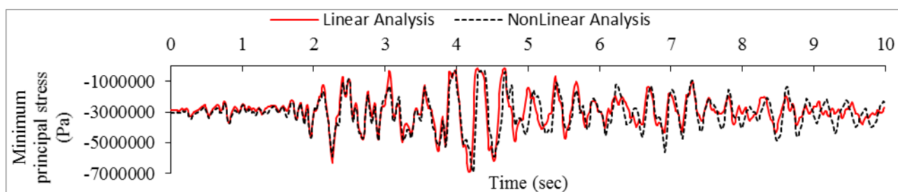
شکل ۱۹: تاریخیچه‌ی زمانی تنش اصلی سوم در محل تراز شکستگی بدنه پایین دست سد
