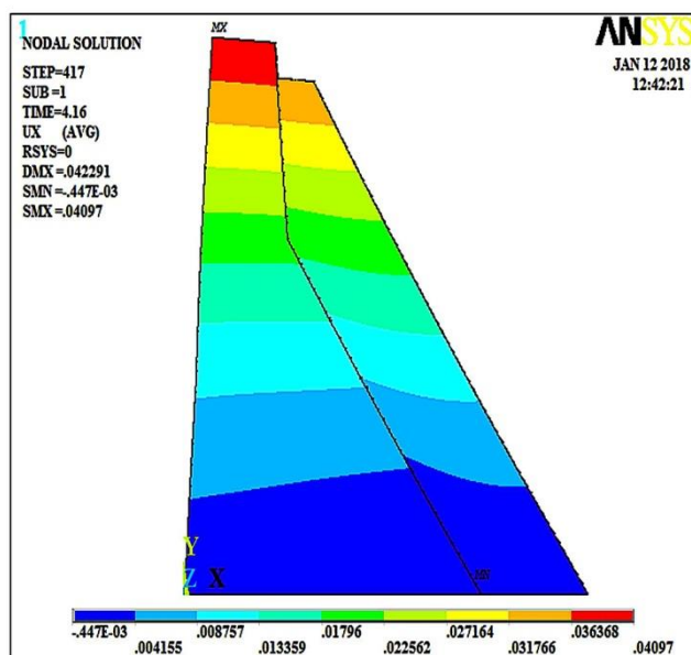
شکل ۲۵: کانتور تغییر مکان قائم سد (t=4.15sec)
