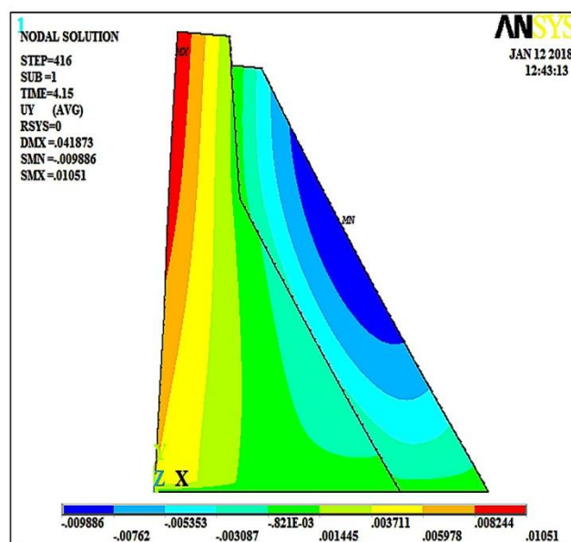
شکل ۲۴: کانتور تغییر مکان افقی سد (t=4.16sec)
