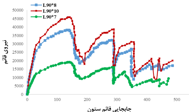
شکل ۱۹: اثر ضخامت بر پاسخ نیرو-جابجایی عمودی اتصال نبشی بالا و پایین
