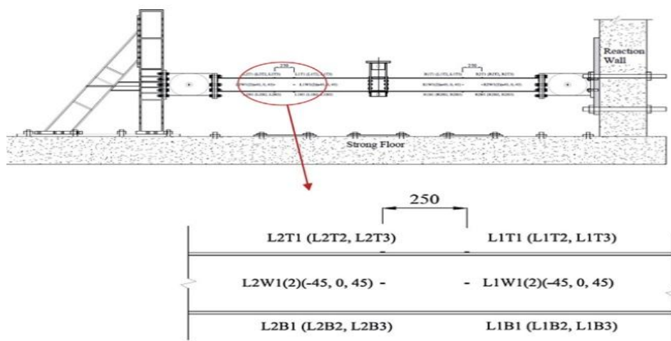
شکل ۵: محل قرارگیری کرنش سنج ها بر روی تیر در آزمایش یانگ وتان [۱۱]
