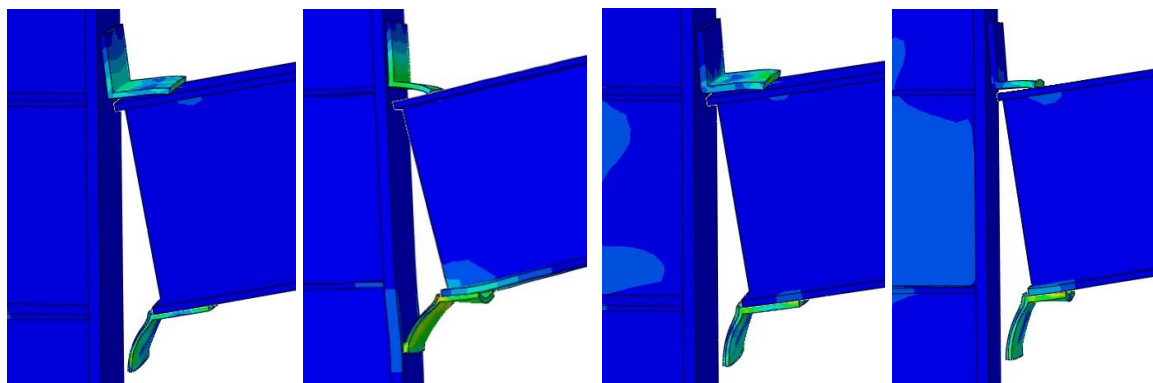
شکل ۲۴: مقایسه مد شکست اتصال نبشی بالا و پایین در اثر استفاده از نبشی با بال نامساوی در نبشی پایین
