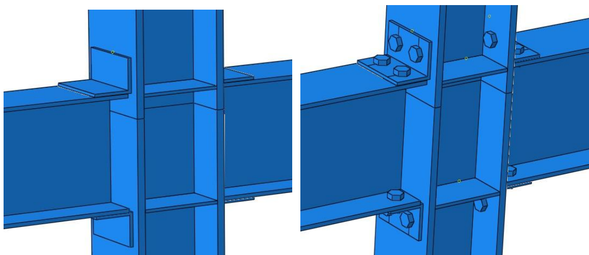
اتصال جوشی
