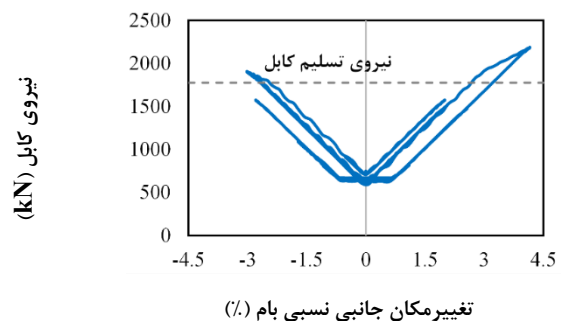
شکل ۸: پاسخ نیرویی کابل‌های پس‌تنیده.
