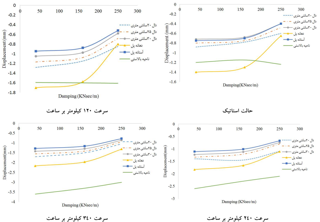
شکل ۱۰: نمودار تغییرات حداکثر تغییر مکان خط در مقایسه با تغییر میرایی خط و سرعت قطار.
