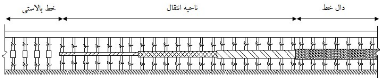
شکل ۳: مدل ناحیه انتقال با پیش دال‌های بتنی بررسی شده توسط ذاکری و همکاران [18].
