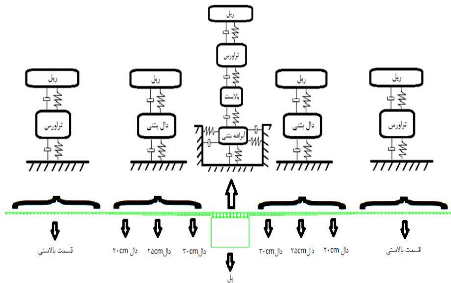
شکل ۱: مدل شماتیک ناحیه انتقال خط بالاستی در محل آبرو بتنی شامل بایپس دال‌های بتنی.
