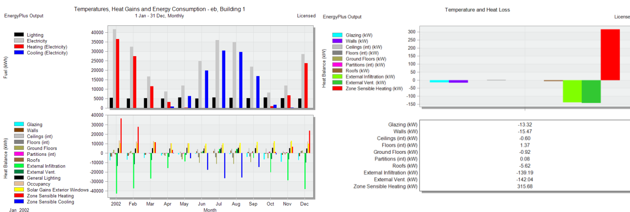
شکل ۴: اتلاف حرارتی جداره ها و جزئیات مصرف انرژی ماهیانه برای ساختمان حالت K.
