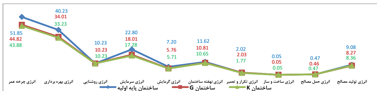
شکل ۵: نمودار مقایسه جزئیات انرژی در ساختمانهای مورد مطالعه (گیگاژول بر مترمربع).
