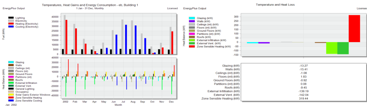
شکل ۳: اتلاف حرارتی جداره ها و جزئیات مصرف انرژی ماهیانه برای ساختمان حالت G.
